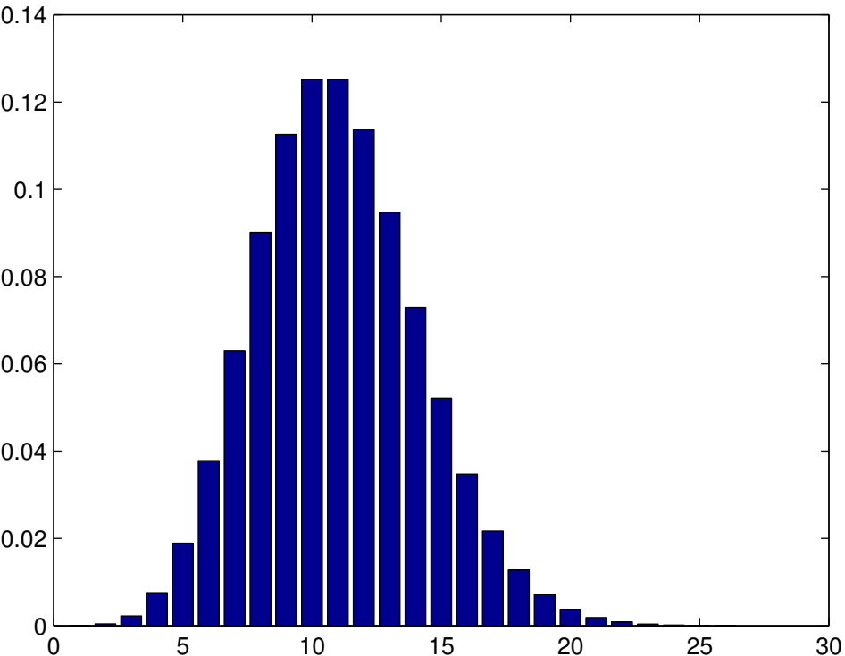
Poi( \lambda=10.000 )
