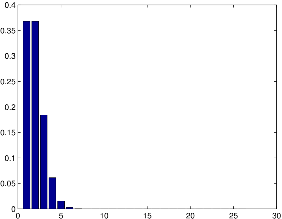
Poi( \lambda=1.000 )
