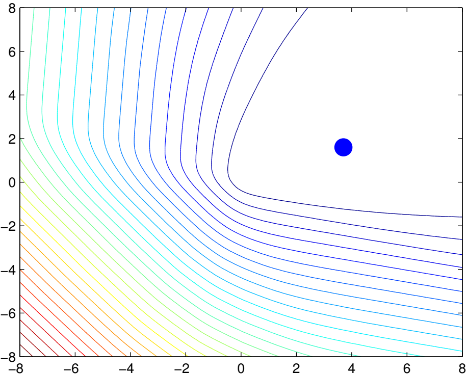
Log-Unnormalised Posterior
