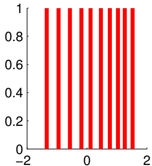
K=10 , mse=0.0111
