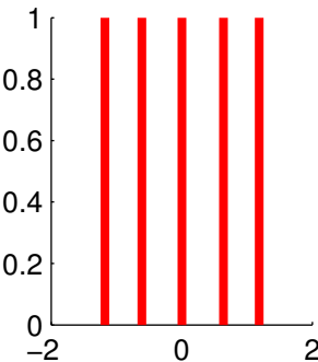
K=5 , mse=0.0368
