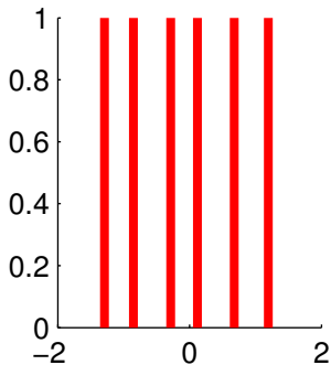
K=6 , mse=0.0275
