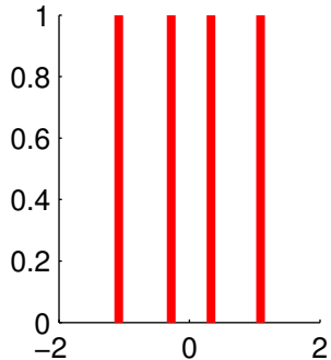
K=4 , mse=0.0562
