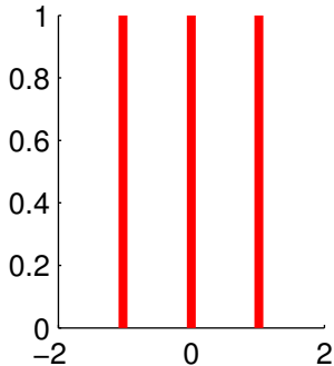
K=3 , mse=0.0818
