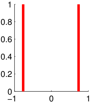
K=2 , mse=0.2023
