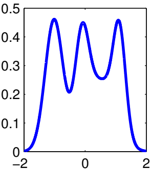
K=5, nll=1202.5869
