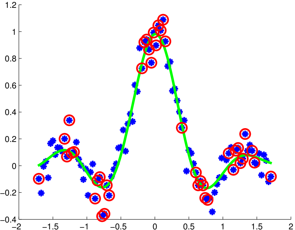
linregL1
