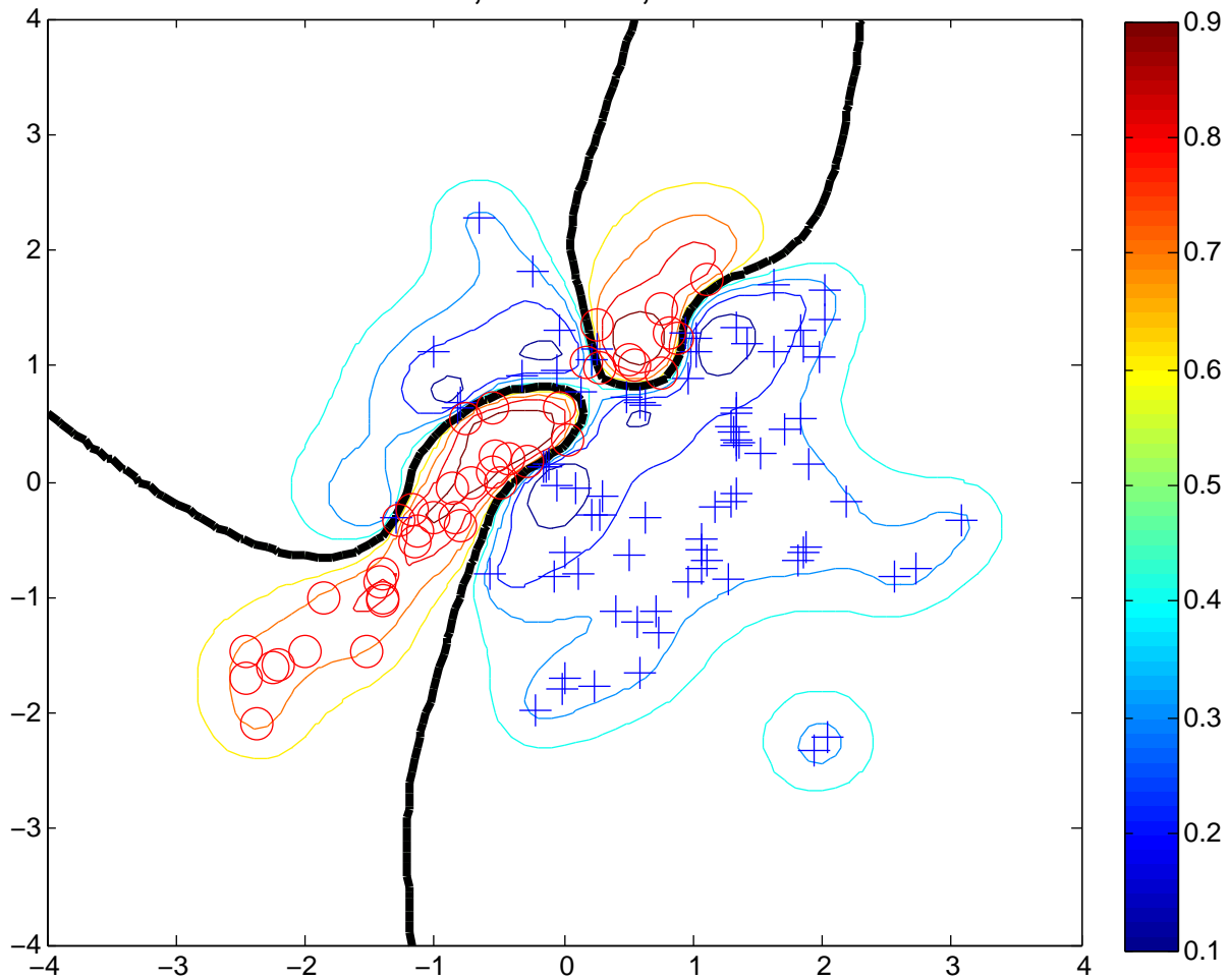
SE kernel, l=0.500 , \sigma^2=10.000
