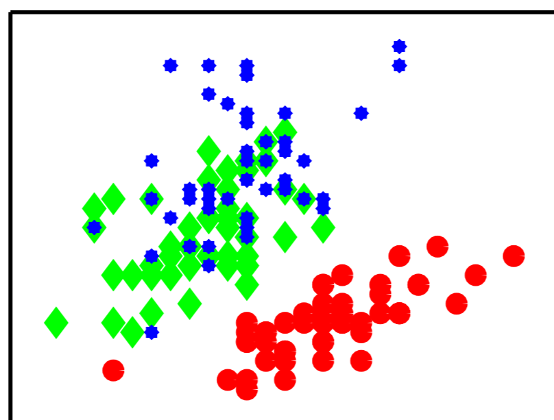
sepal width
