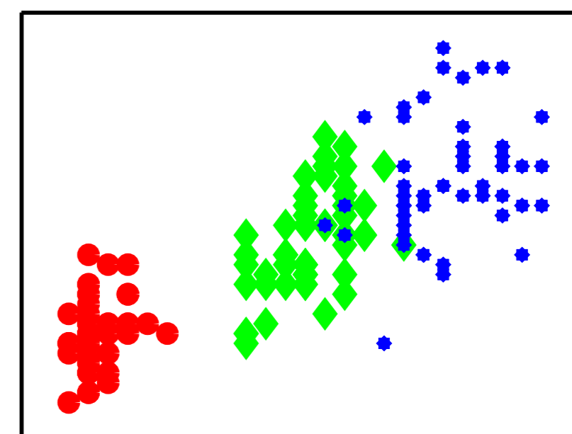
petal width
