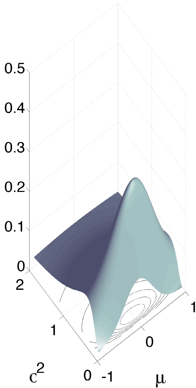
NIX( \mu_0=0 , k_0=1 , v_0=1 , c_0^2=1 )
