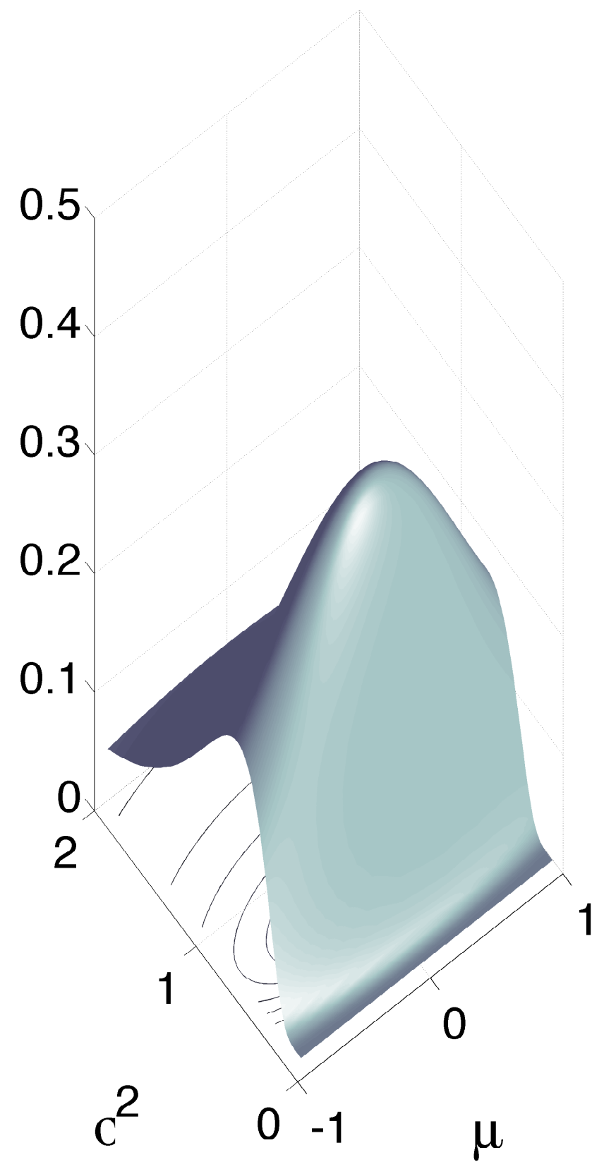
NIX( \mu_0=0 , k_0=1 , v_0=5 , c_0^2=1 )
