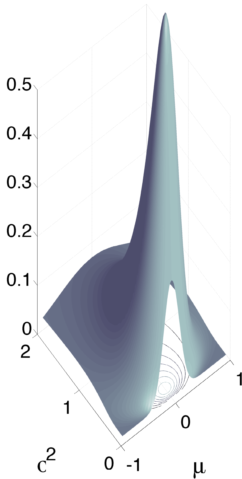
NIX( \mu_0=0 , k_0=5 , v_0=1 , c_0^2=1 )
