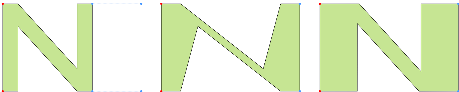
Input
