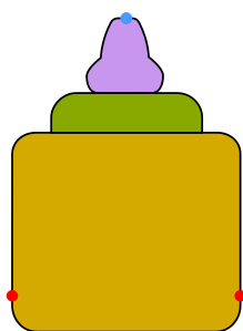
Ours
