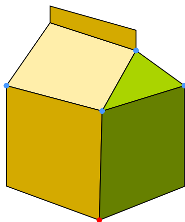
Ours
