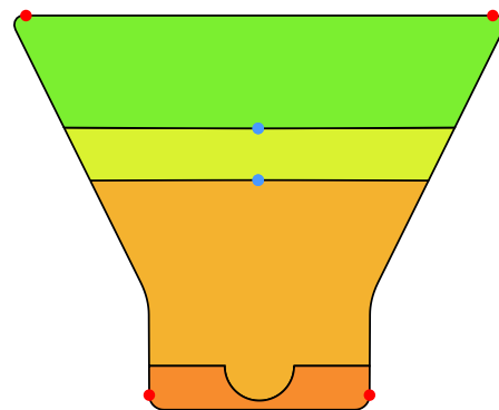
Ours
