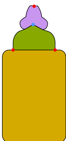
Poisson
