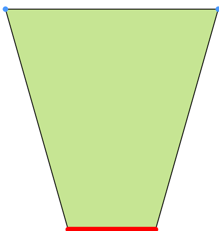
Poisson
