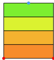
Ours
