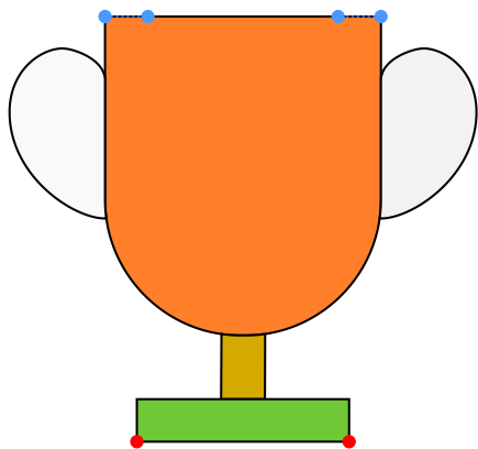
Input
