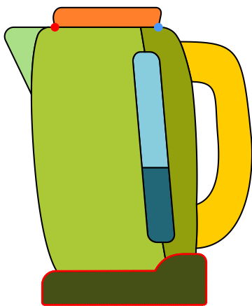
Poisson
