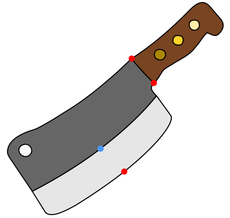
Ours
