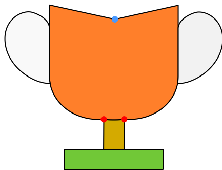
Poisson
