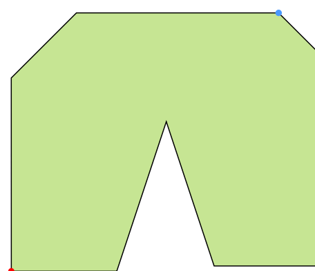
Ours
