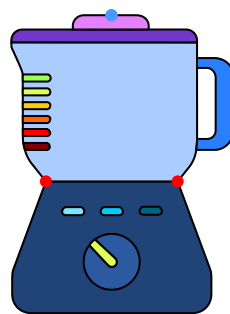
Ours
