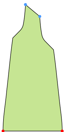
Ours
