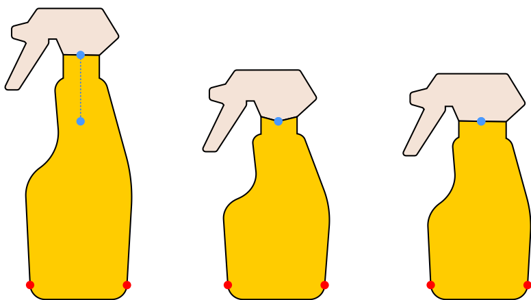
Input
