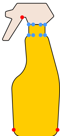
Input
