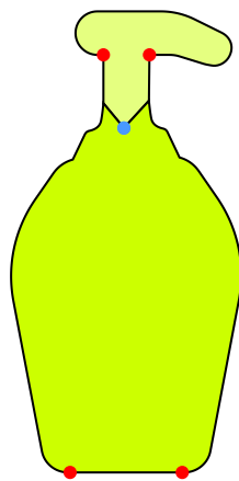
Poisson
