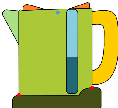
Poisson
