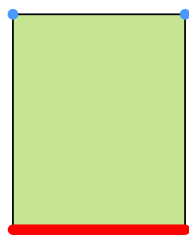
Ours
