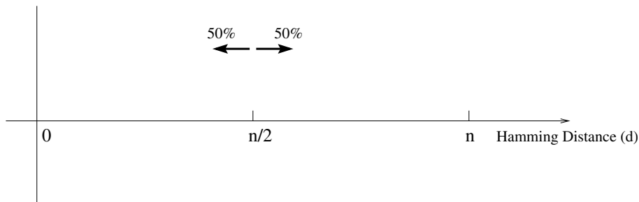
Fig. 1. A Random Walk
